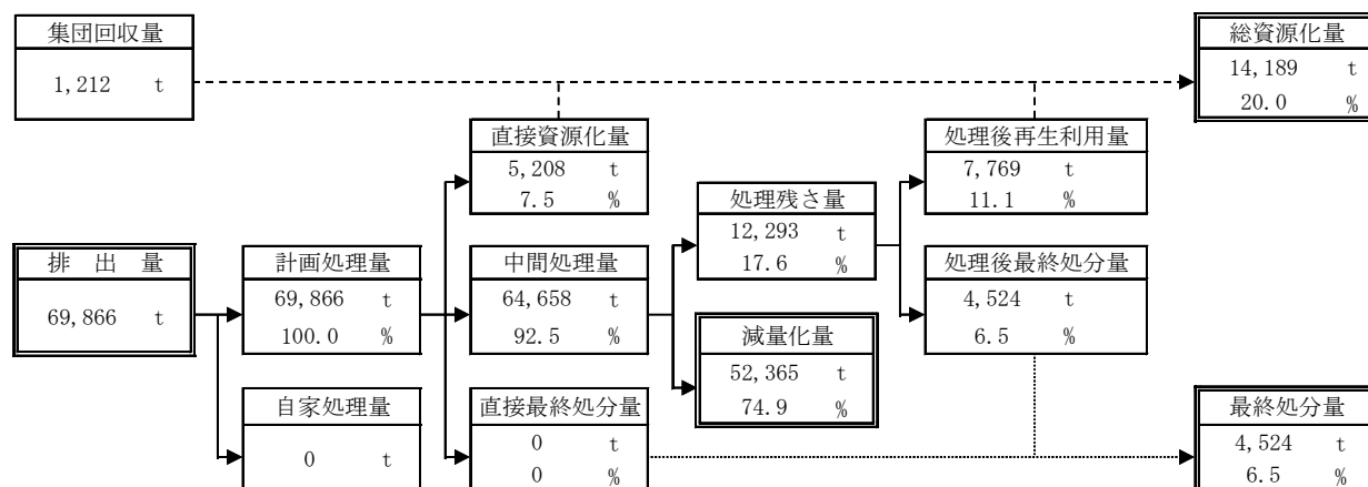
図 2 一般廃棄物の処理状況フロー（平成 30 年度）
