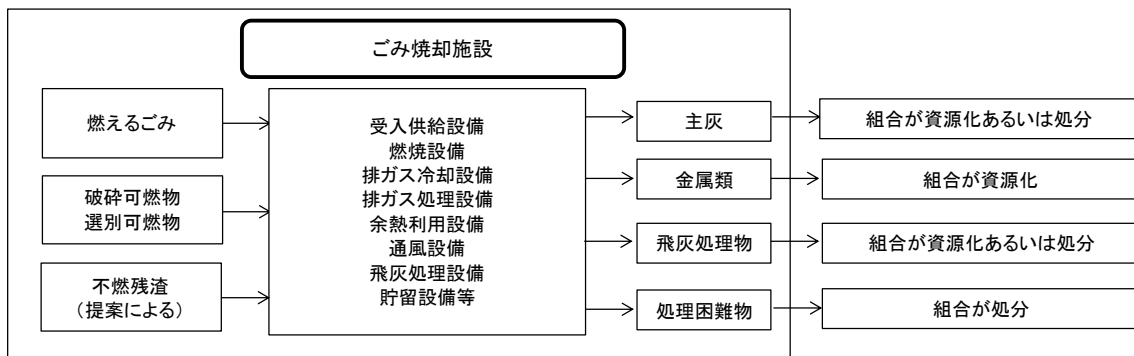
図 ごみ焼却施設の処理フロー(主灰の処理を外部委託する場合)(案)
