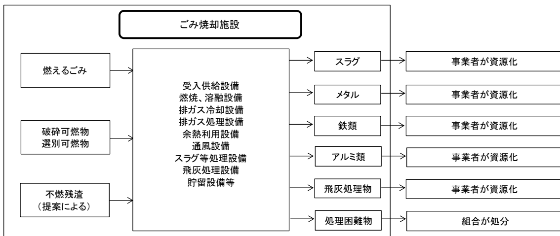
図 ごみ焼却施設の処理フロー(熔融処理を行う場合)(案)
