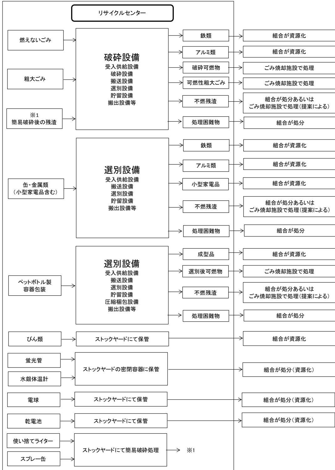
図 リサイクルセンターの処理フロー(案)
